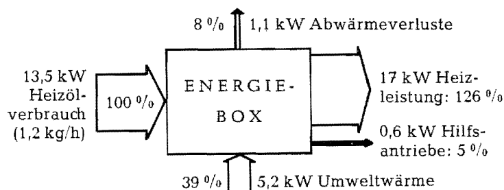
Bild 2: Energieflüsse bei der Energiebox mit integrierter Wärmepumpe
