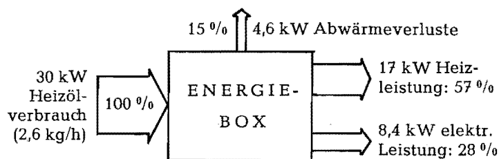
Bild 1: Energieflüsse bei der Energiebox
